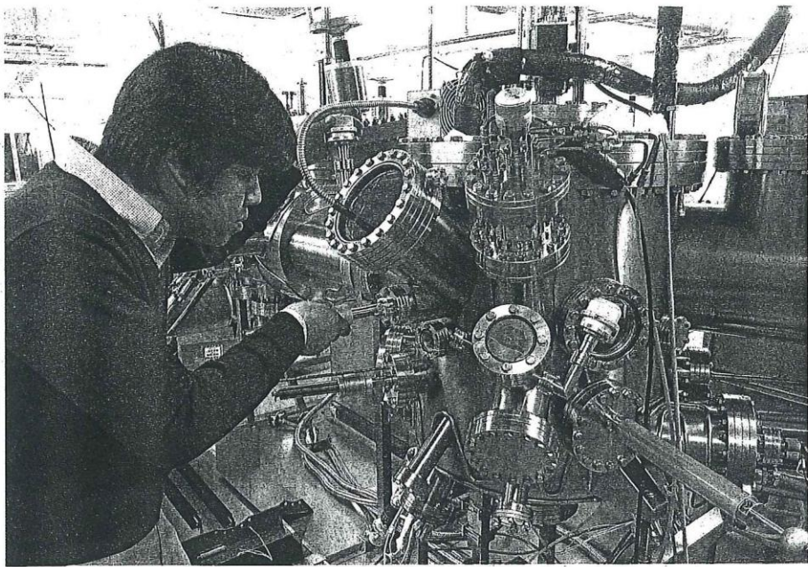
シリコンとゲルマニウムを組み合わせた結晶を作る「シリコン分子線エピタキシー装置」 10月30日、東京都世田谷区の東京都市大
